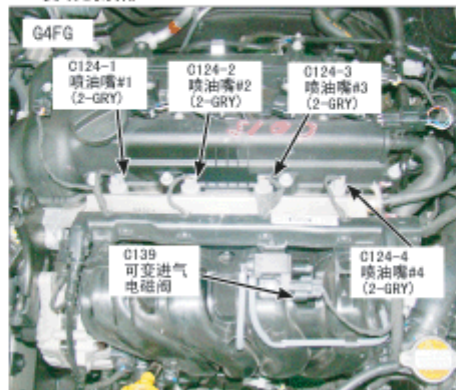
17. 发动机顶部
