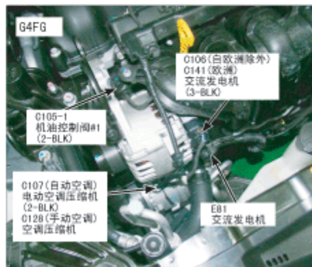
14. 发动机前右
