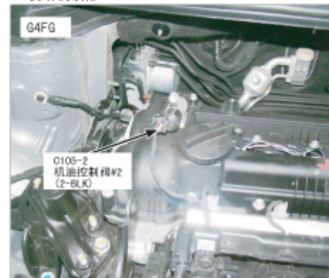
18. 发动机顶部
